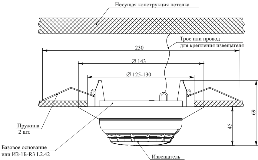
Рисунок А.2 – Установка извещателя на подвесном потолке с базовыми основаниями W2.02, W2.03 или ИЗ-1Б-Р3 L2.42
